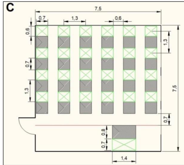
Fig. C – banchi da 70 x 70 cm (scuola secondaria di I° e II° grado), con finestre a bascula con apertura in alto.
