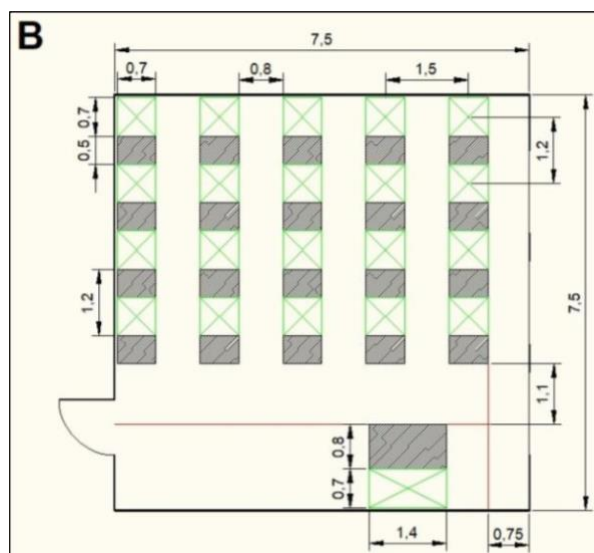
Fig. B – banchi da 70 x 50 cm (scuola secondaria di I° e II° grado), con finestre a bandiera verso l'interno (ante da 0,7 m);
